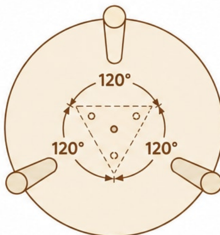
Vista inferior del tablero
