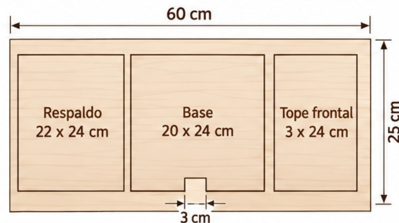
Plano de corte (tablero de 60 x 25 cm)
