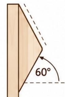
Detalle del corte en ángulo (60°)
